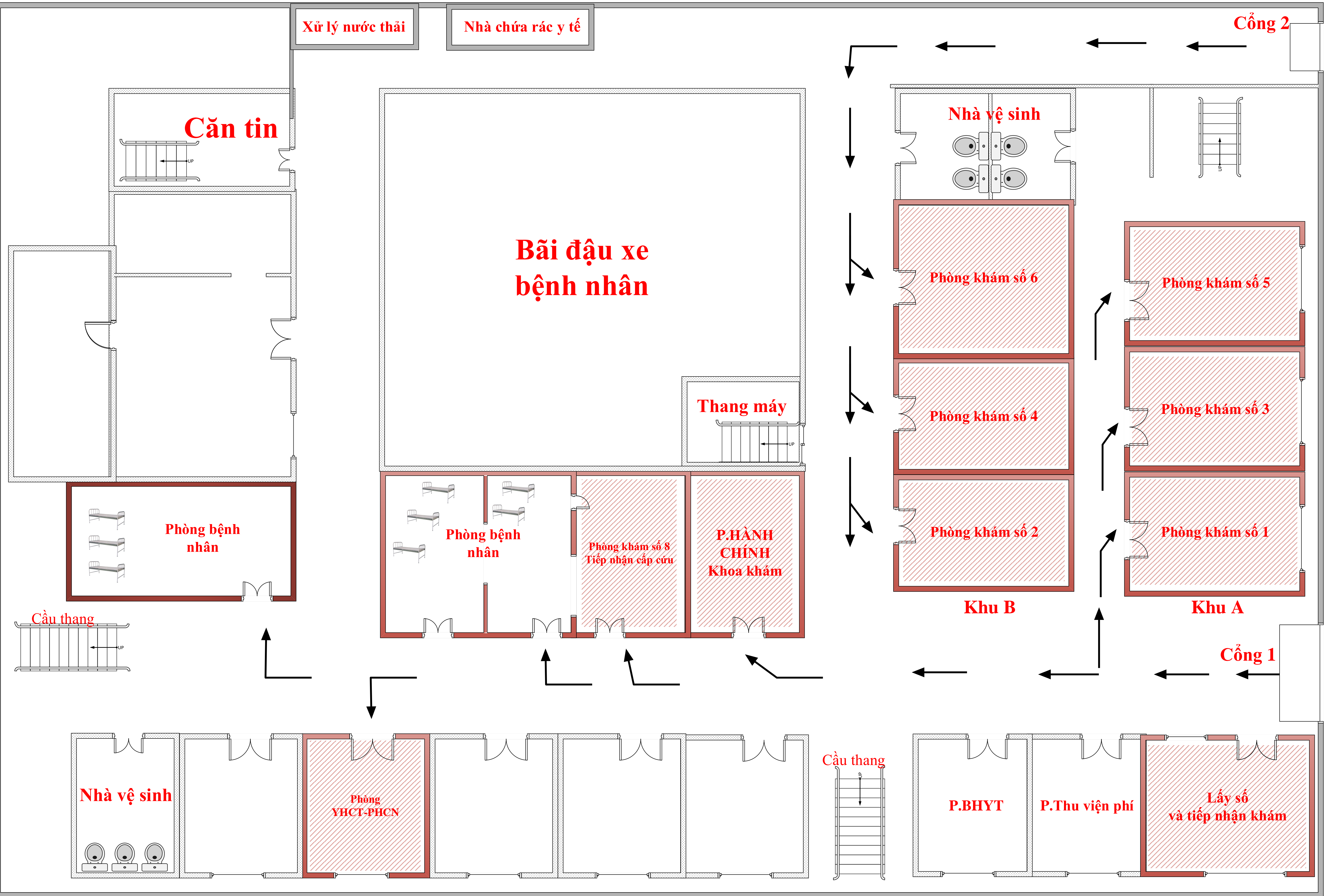
SƠ ĐỒ KHOA KHÁM BỆNH - CẤP CỨU TẦNG TRỆT
